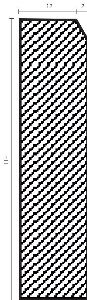
Musterquerschnitt
